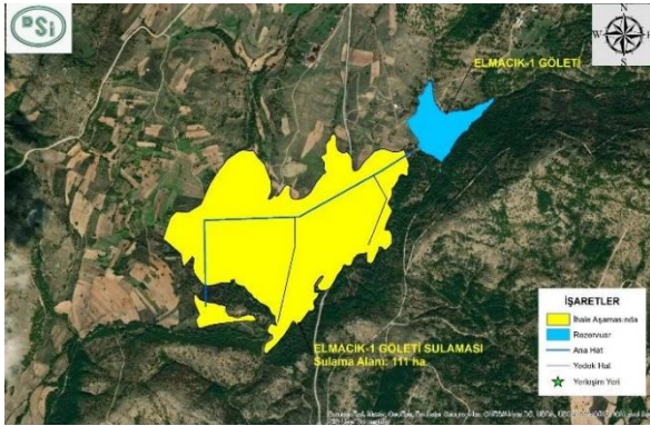
Kofçaz Elmacık 1 Göleti
